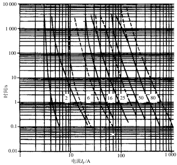
图 A.1 熔断器熔丝的时间-电流区域
