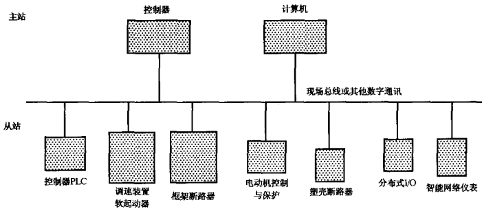
图1 系统配置
